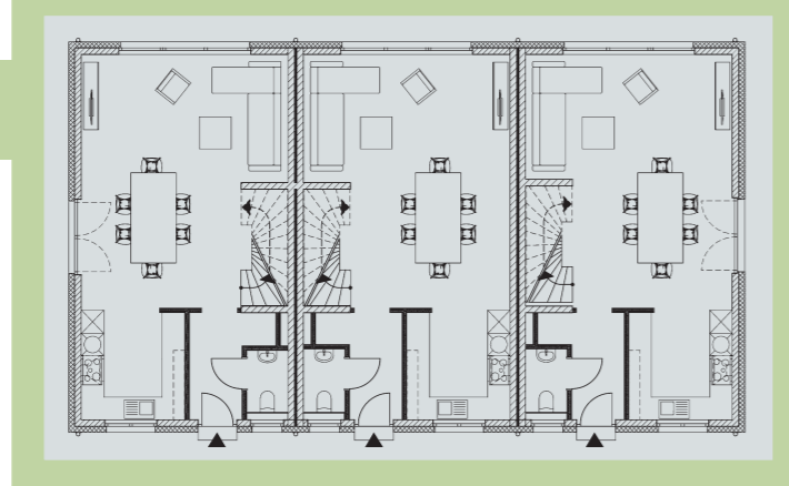
Beispiele für Erdgeschoss-Grundrisse Reihenhaus-Standardvariante
